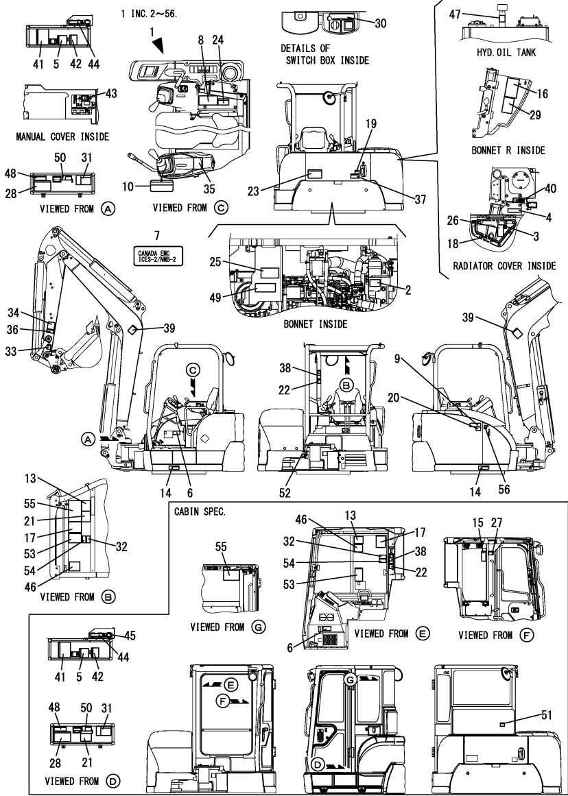
Fig.200. LABEL KIT(FOR CANADA)(OPTIONAL)
