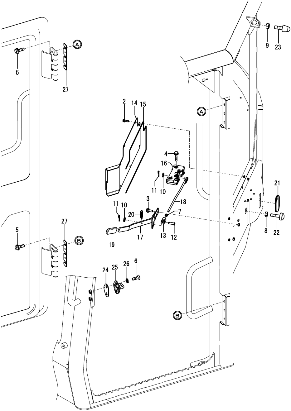
Fig.105. CABIN DOOR(1)
