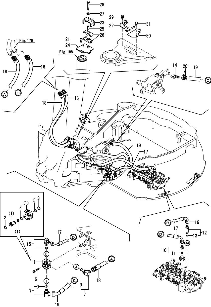
Fig.175. P.T.O.(CONTROL VALVE - BOOM)
