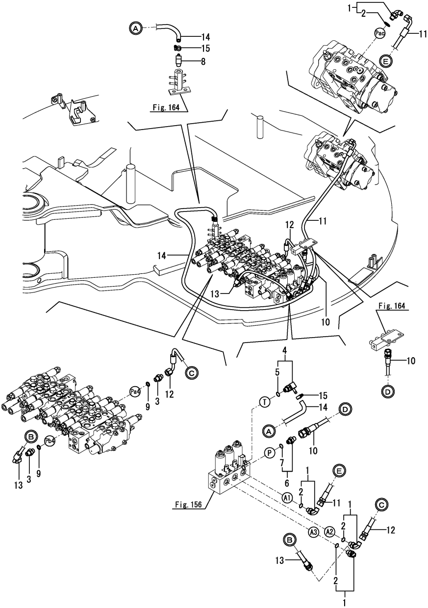
Fig.179. P.T.O.(SOLENOID VALVE & E.S.S.)
