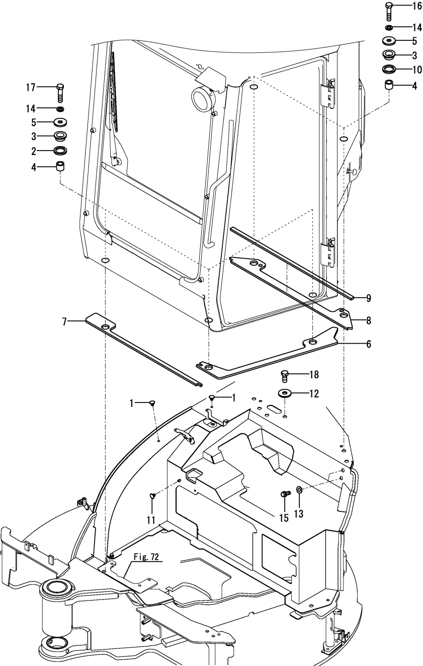
Fig.114. CABIN(PAD)
