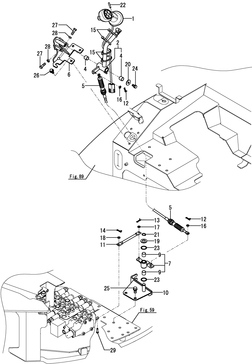
Fig.66. BLADE LEVER(ANGLE BLADE SPEC.)
