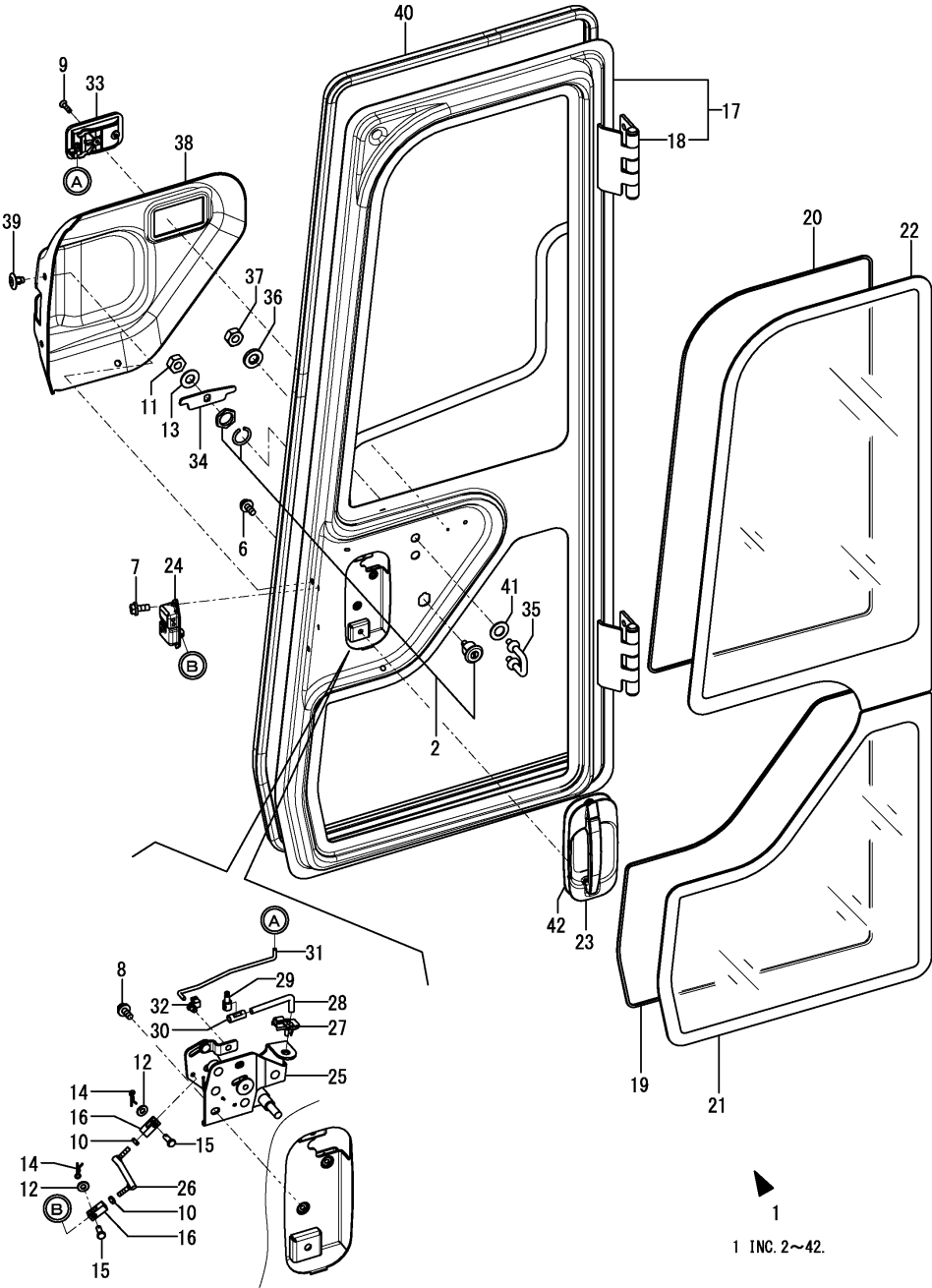
Fig.106. CABIN DOOR(2)
