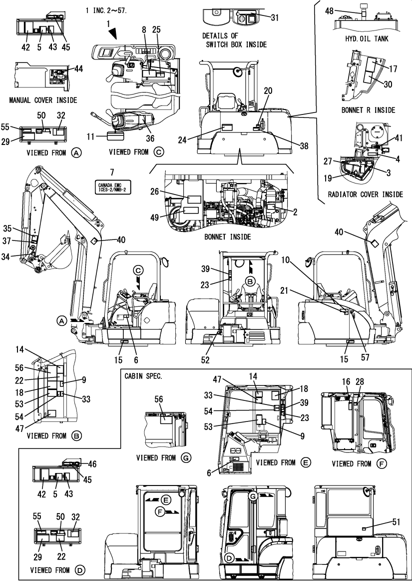
Fig.201. LABEL KIT(FOR CANADA)(ANGLE BLADE SPEC.)(OPTIONAL)
