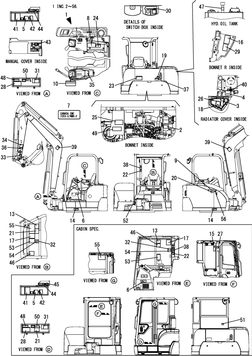
Fig.200. LABEL KIT(FOR CANADA)(OPTIONAL)
