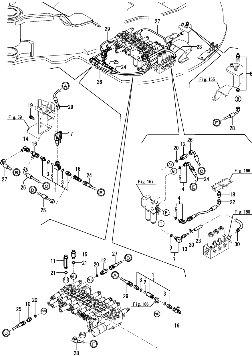
Fig.181. P.T.O.2(ANGLE BLADE SPEC.)
